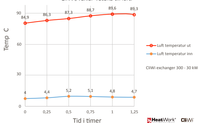
HeatWork lyfter temperaturer upp till 90°C med CliWi CliWi, växlar vätska till luft.
